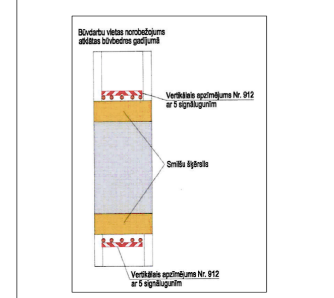
SATIKSMEŠ ORGANIZĀCIJA DARBU VIETĀ - VARIANTS NR. 5
