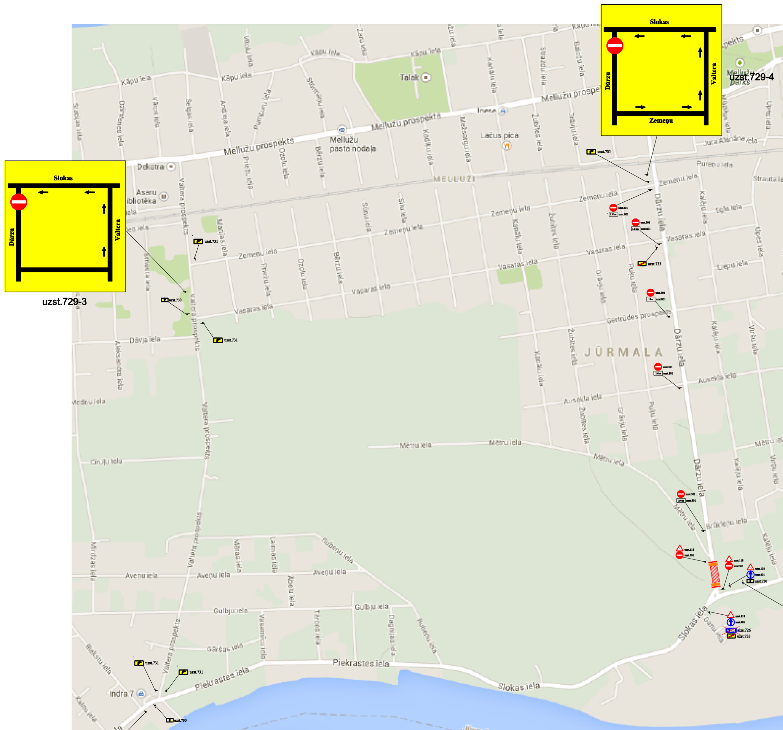
SATIKSMEŠ ORGANIZĀCIJA DARBU VIETĀ - VARIANTS NR. 5
